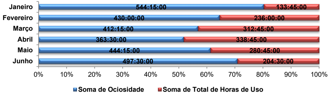
Evolução da Relação Entre Ociosidade e Horas Mensais de Uso, do Espectrômetro de 4,7 Tesla, no Período de Janeiro a Junho de 2024
