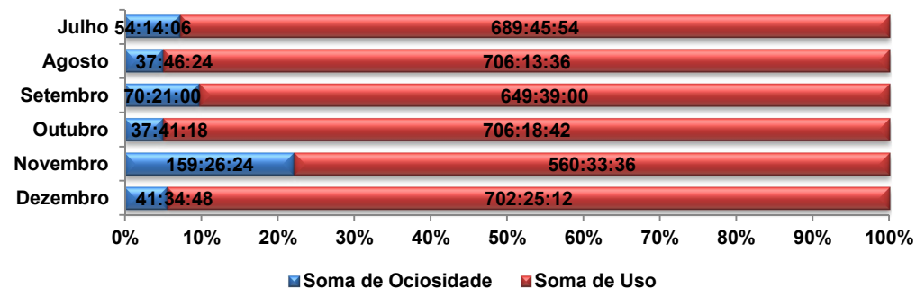
Relação Entre Ociosidade e Horas de Uso, do Espectrômetro de 9,4 Tesla, no Período de Julho a Dezembro de 2024
