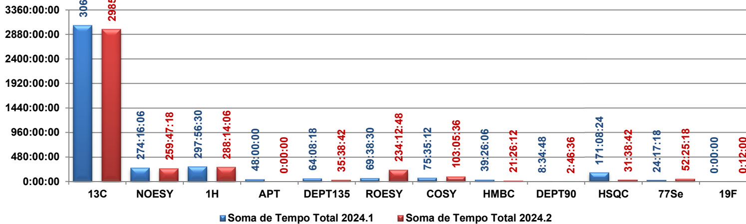
Total de Horas de Uso do Espectrômetro de 9,4 Tesla, por Tipo de Experimento, nos Períodos de Janeiro a Junho e Julho a Dezembro de 2024
