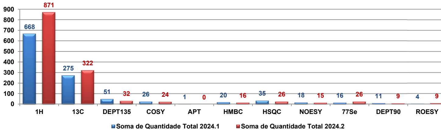
Tipos de Experimentos Realizados e Respectiveas Quantitativos, no Espectrômetro de 9,4 Tesla nos Períodos de Janeiro a Junho e Julho a Dezembro de 2024
