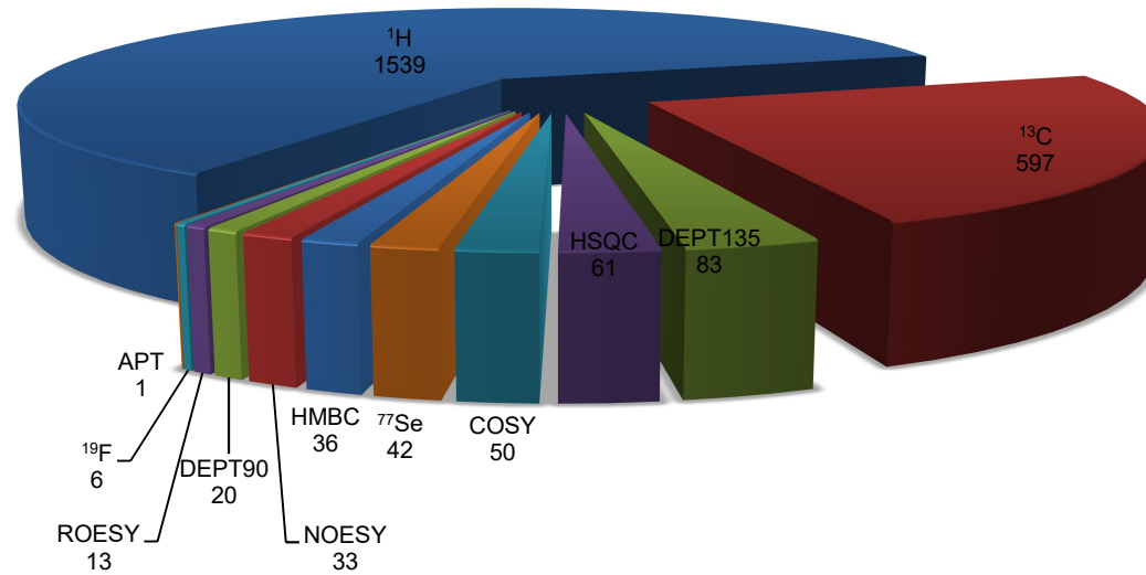
Tipos de Experimento e Respectiveas Quantidades, Realizados Pelo Espectrômetro de 9,4 Tesla, no Ano de 2024
